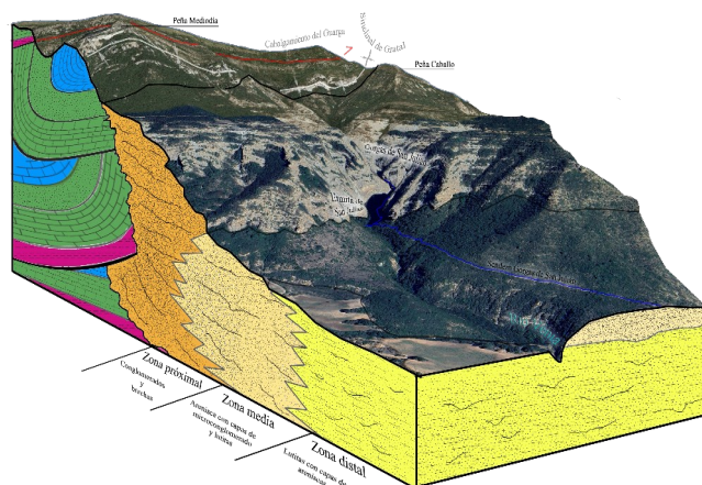
Esquema geológico de las Gorgas
